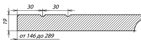
Сечение ПСЯ
