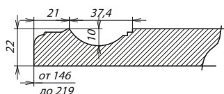
Сечение ПСЯ
