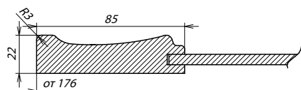
Сечение фасада
