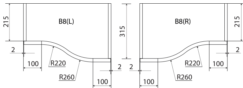
ВЕРХНИЙ МОДУЛЬ С S - ОБРАЗНЫМ ФАСАДОМ B8 МИН./МАКС ВЫСОТА, ММ: 496/1000
