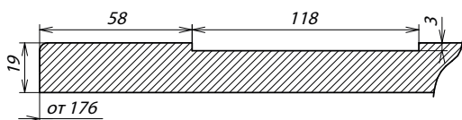
Сечение фасада
