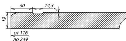
Сечение ПСЯ
