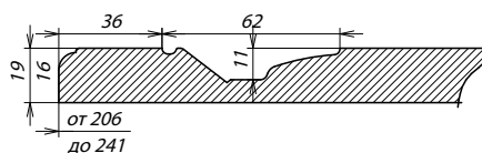
Сечение ПСЯ
