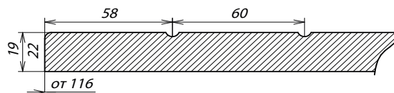
Сечение фасада
