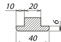
Планка стыковочная
