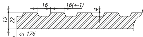
Сечение фасада
