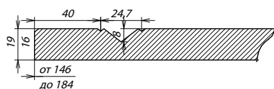
Сечение ПСЯ
