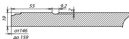
Сечение ПСЯ
