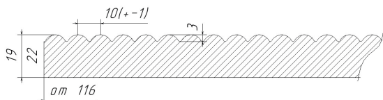
Сечение фасада
