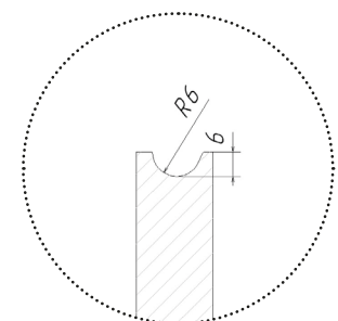
LINE MINI
