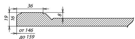
Сечение ПСЯ
