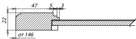
Сечение фасада
