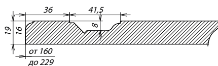
Сечение ПСЯ
