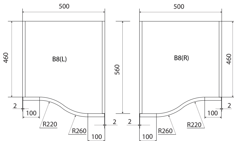
НИЖНИЙ МОДУЛЬ С S - ОБРАЗНЫМ ФАСАДОМ B8 МИН./МАКС ВЫСОТА, ММ: 496/1000
