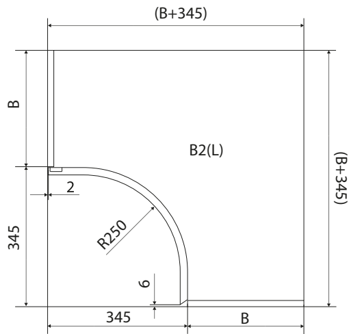
НИЖНИЙ МОДУЛЬ С ВОГНУТЫМ ФАСАДОМ B2(L/R) B2(L) - ЛЕВЫЙ, B2(R) - ПРАВЫЙ, В ЗАВИСИМОСТИ ОТ ОТКРЫВАНИЯ, НА ЭСКИЗЕ ПРЕДСТАВЛЕН B2(L) МИН./МАКС ВЫСОТА, ММ: 496/960
