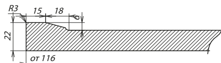
Сечение фасада
