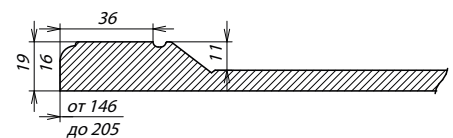
Сечение ПСЯ
