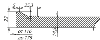
Сечение ПСЯ
