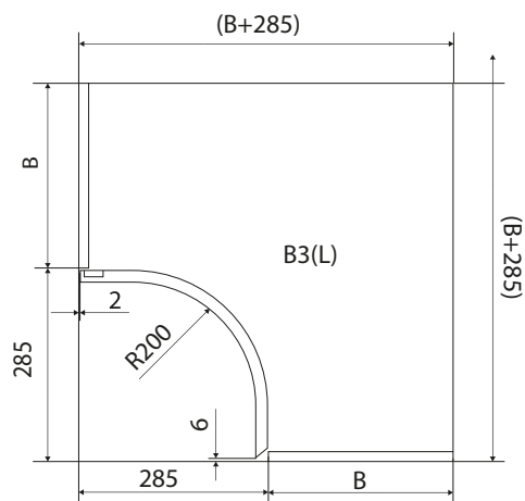
ВЕРХНИЙ МОДУЛЬ С ВОГНУТЫМ ФАСАДОМ B3(L/R) B3(L) - ЛЕВЫЙ, B3(R) - ПРАВЫЙ, В ЗАВИСИМОСТИ ОТ ОТКРЫВАНИЯ, НА ЭСКИЗЕ ПРЕДСТАВЛЕН B3(L) МИН./МАКС ВЫСОТА, ММ: 496/1600
