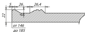
Сечение ПСЯ
