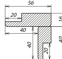
Угловое соединение торцевых планок
