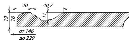
Сечение ПСЯ
